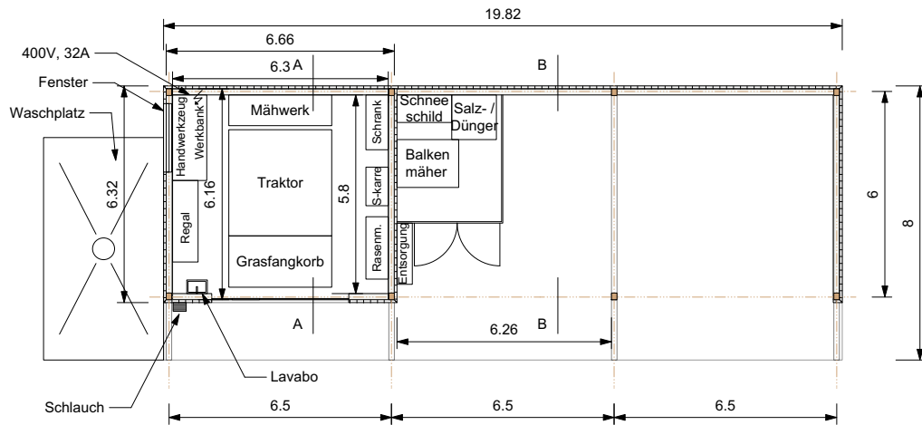
Grundriss
